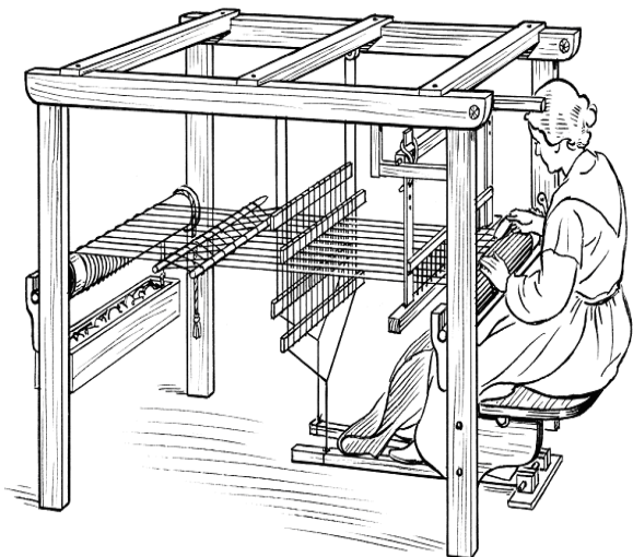
Schéma ručního tkalcovského stavu
