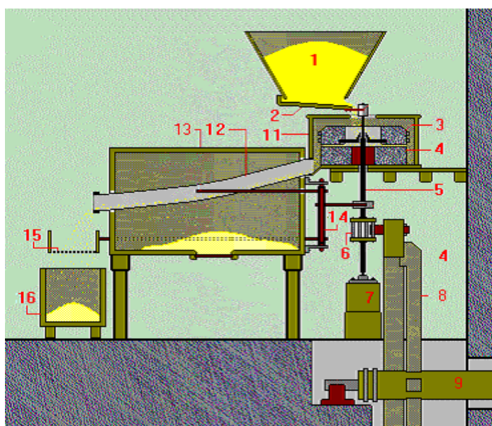
Schéma starého českého mlýna s obvyčejným mlecím složením
